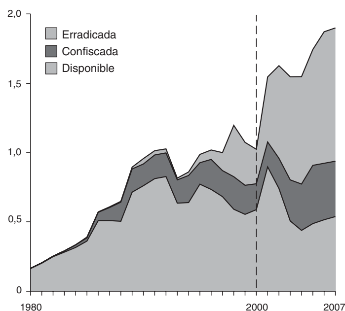
GRÁFICA 15 Cocaína sin las medidas antidrogas
